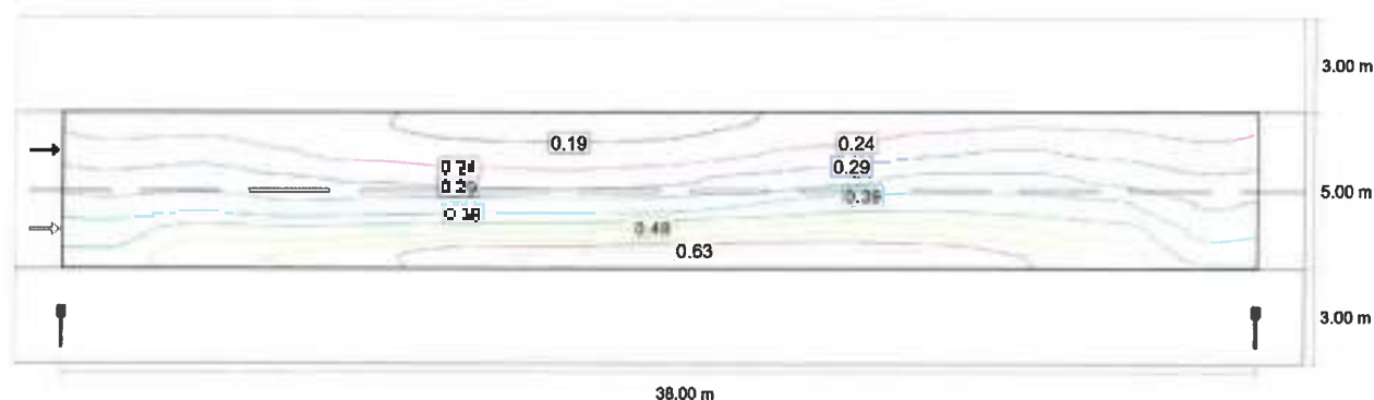
Observator 2: Valoarea de întreținere, densitatea lumini cu carosabil uscat ( cd/m^2 ) (Linii Isolux)
