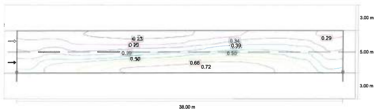
Observator 1: Valoarea de întreținere, densitatea lumii cu carosabil uscat [ cd/m^2 ] (Levi (soluș))
