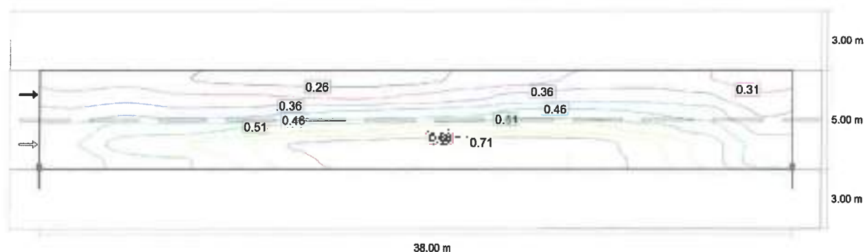
Observator 2: Valoarea de înmăgănire, densitatea luminii cu carosabil uscat [ cd/m^2 ] (Linia 1 sol. ix)
