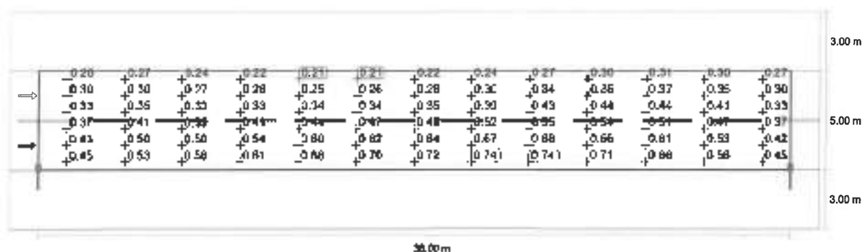
Observator 1: Valoarea de întreținere, densitatea lumii cu carosabil uscat [ cd/m^2 ] (Răster valoric)
