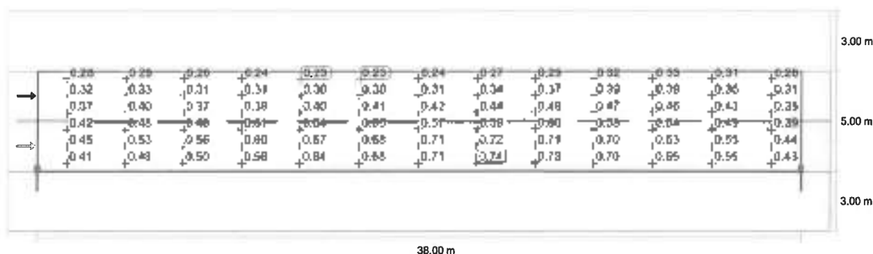
Observator 2: Valoarea de înmăgănire, densitatea luminii cu carosabil uscat [ cd/m^2 ] (Răster valori)
