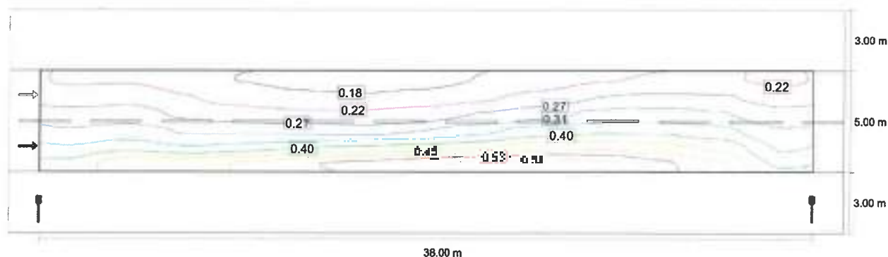
Observator 1: Valoarea de întreținere, densitatea lumini cu carosabil uscat [ cd/m^2 ] (Linii Isolux)
